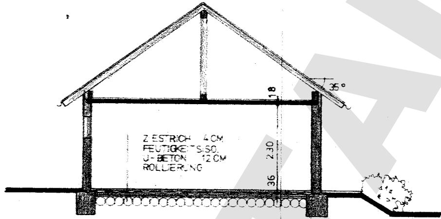
SCHNITT A-A
