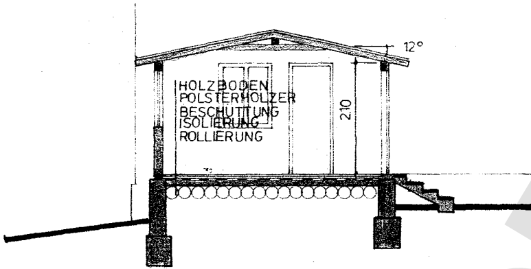
SCHNITT I B-B
